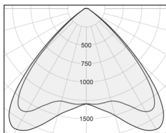
TOP, med optik CEW, for ekstra bredstrålet lysfordeling
