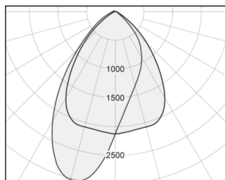
TOP, med optik CRA, for asymmetrisk lysfordeling
