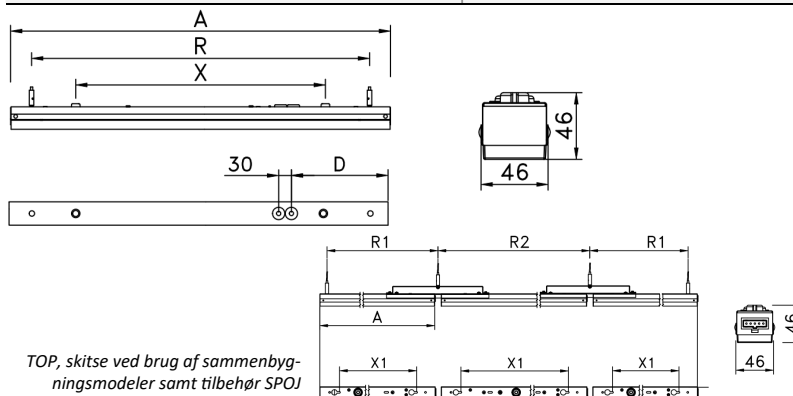
TOP, med optik CRA, for asymmetrisk lysfordeling
