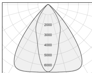
TOP, med optik CHR, for reolgange
