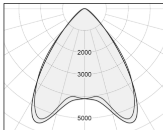
TOP, med optik CW, for bredstrålet lysfordeling
