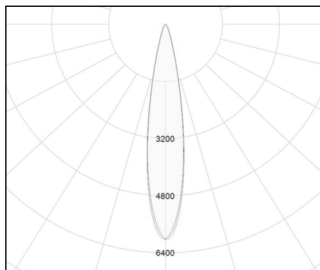
EVO, smalstrålet optik 30°
