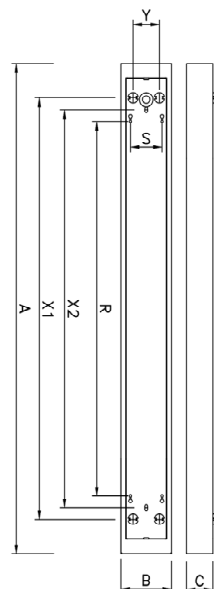
EVO, asymmetrisk optik
