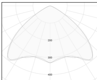
EVO, Ekstra bredstrålet optik 110°
