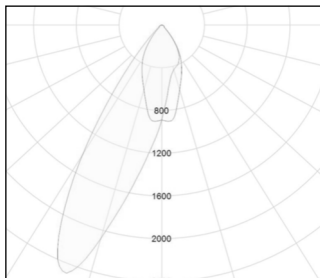
EVO, asymmetrisk optik
