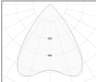
EVO, bredstrålet optik 60°
