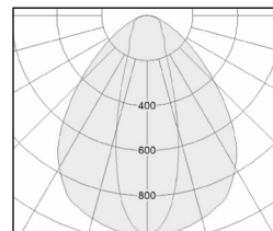
TIP, med optik CHR, for lysfordeling til reolange
