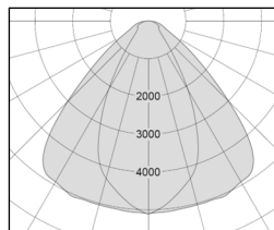
TIP, med optik CN, for smalstrålet lysfordeling
