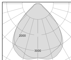
TIP, med optik CW, for bredstrålet lysfordeling
