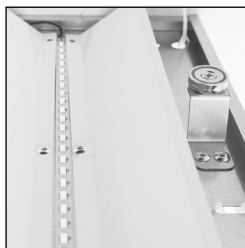
ID, som påbyg, kraftig magnetholder af armaturtop, gør armaturet nemt at montere og uden synlige monterings-skruer
